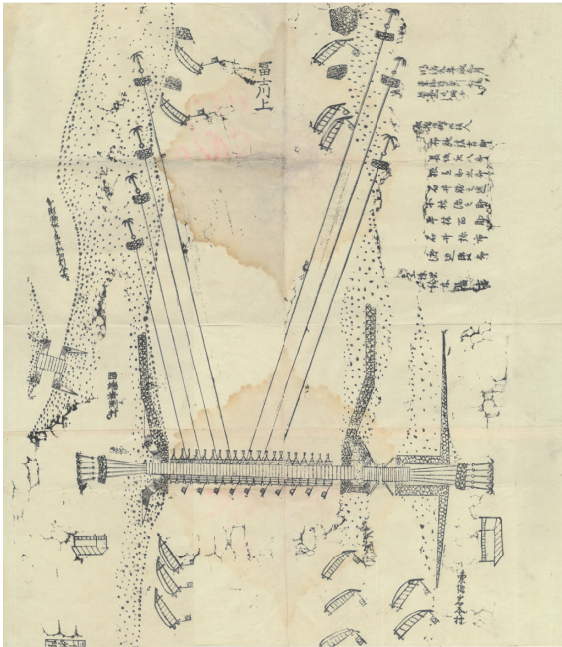
図2：明治元年辰九月東海道富士川船橋四百分一之略図
